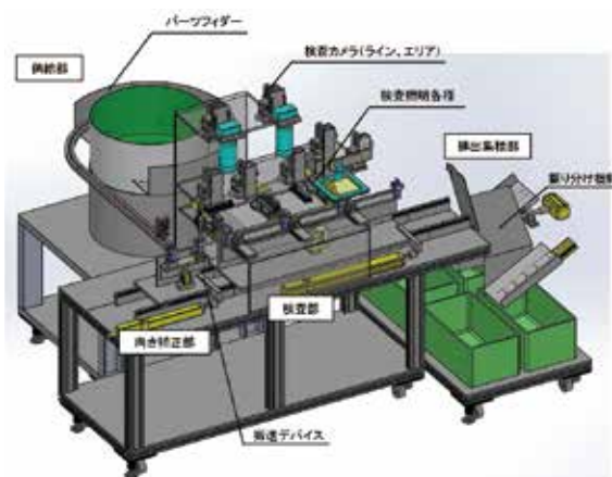
加工鋼管自動外観検査機
