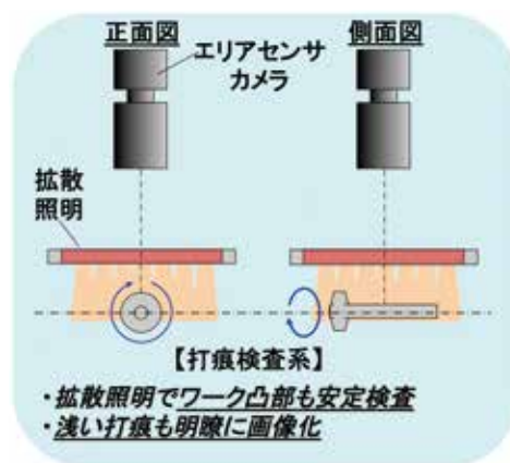
打痕検査装置例
