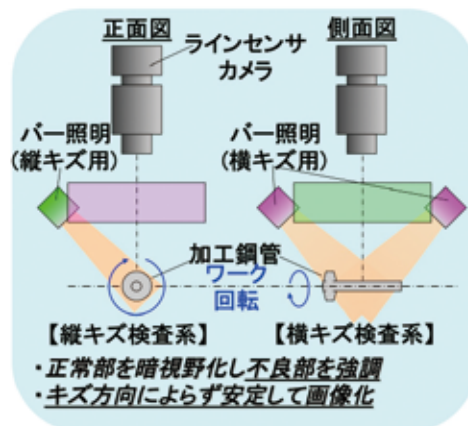
キズ検査装置例
