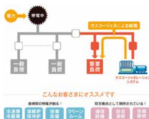
停電時再給電システム概要
