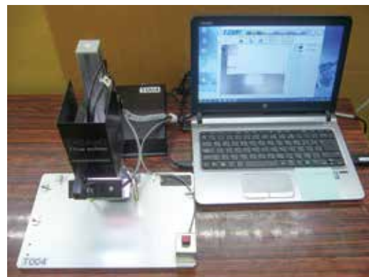
画像検査システム
